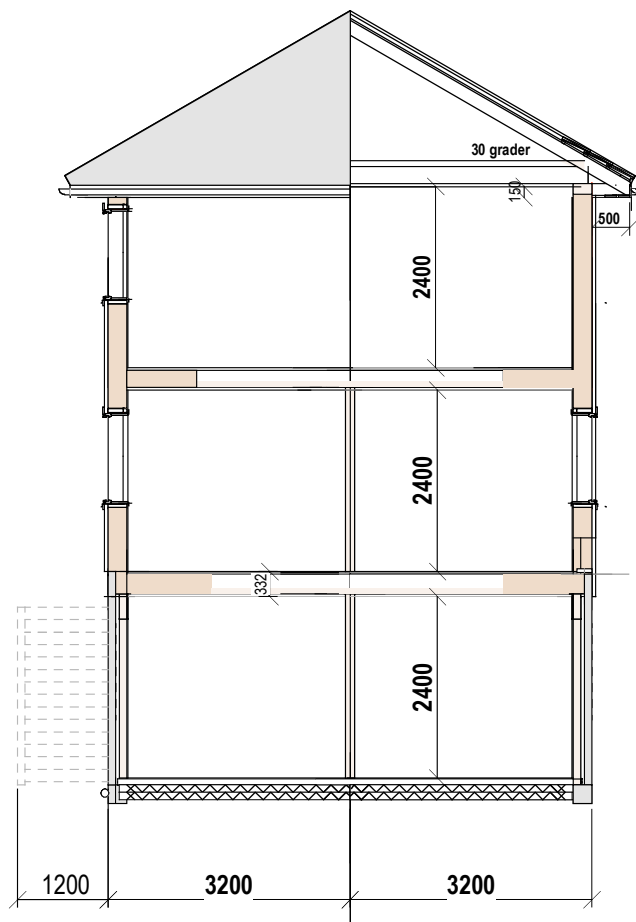
Snitt
