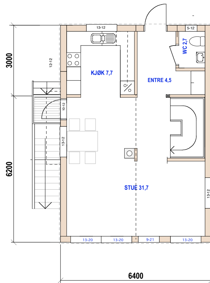
1. Etg.
