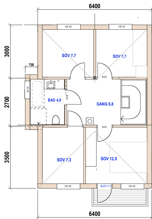
2. Etg.
