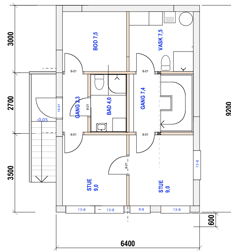
U. Etg.
