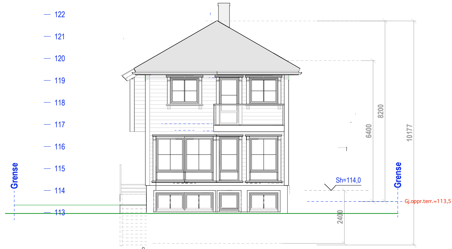
Hus 5 SYD
