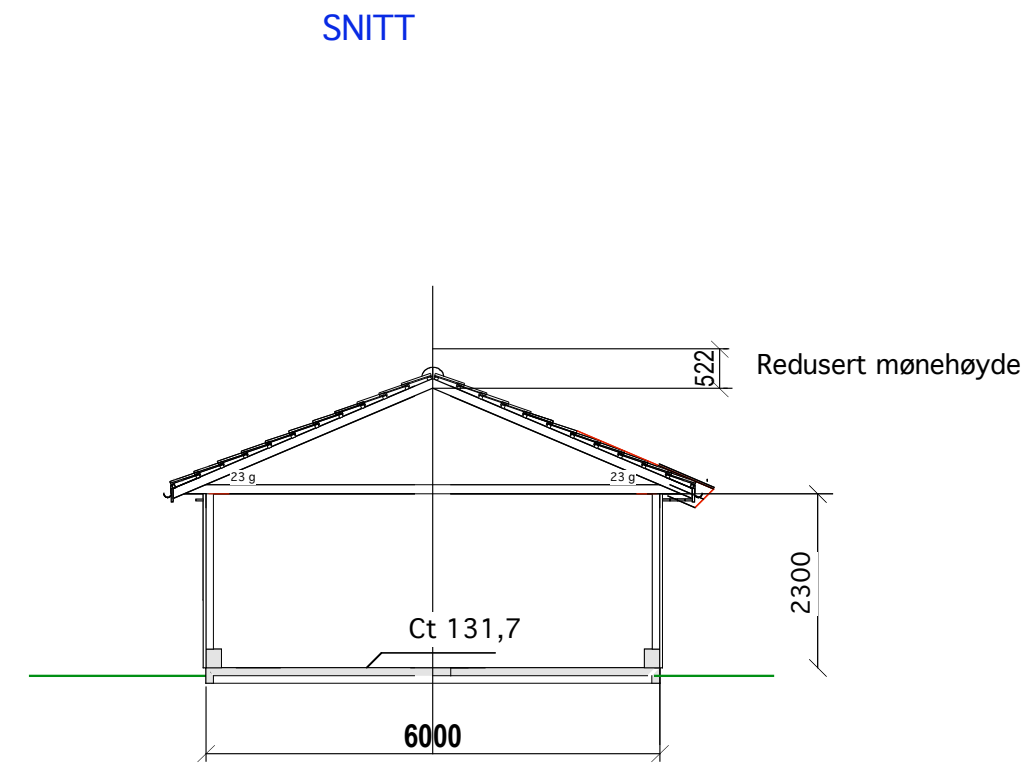
SNITT CP 1
