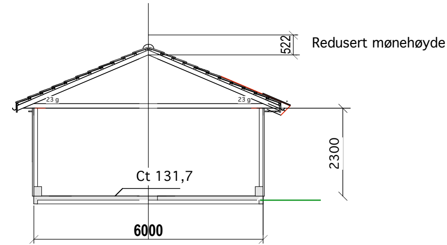
SNITT CP 2
