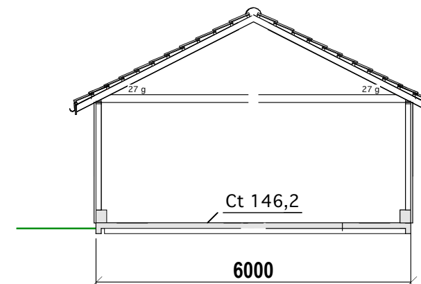
SNITT
