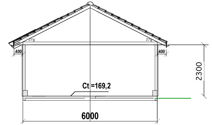
SNITT
