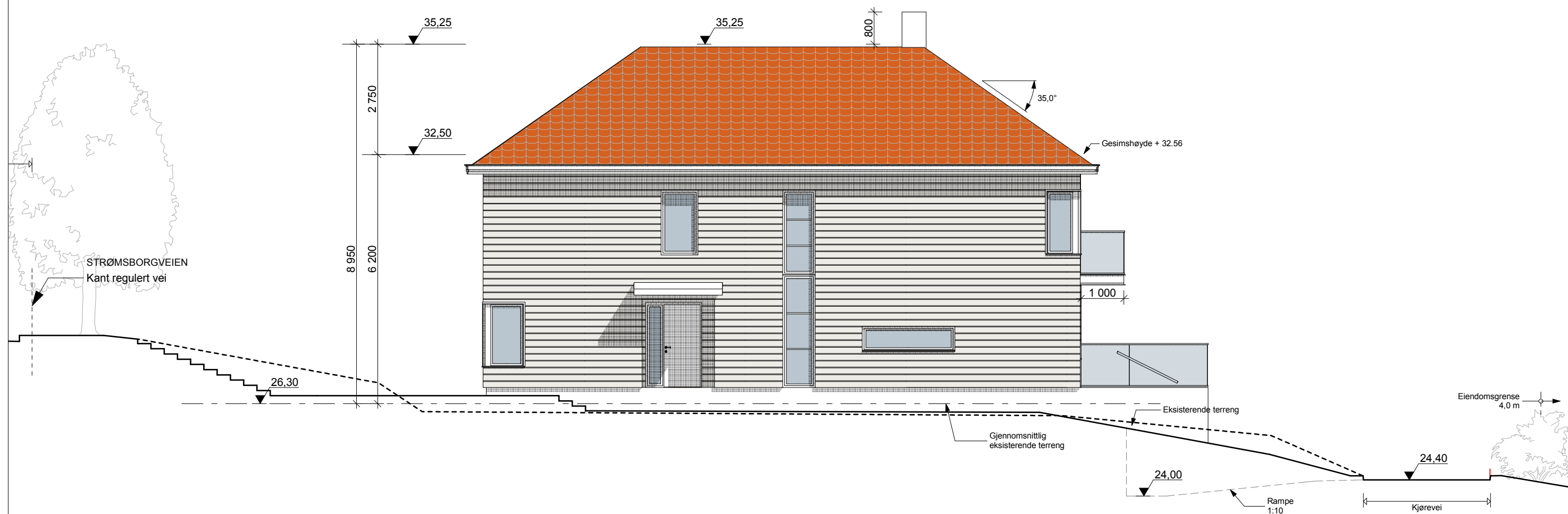
FASADE NORD HUS B MOT EKSISTERENDE BOLIG
