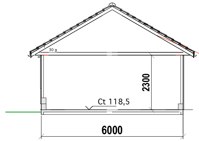
SNITT
