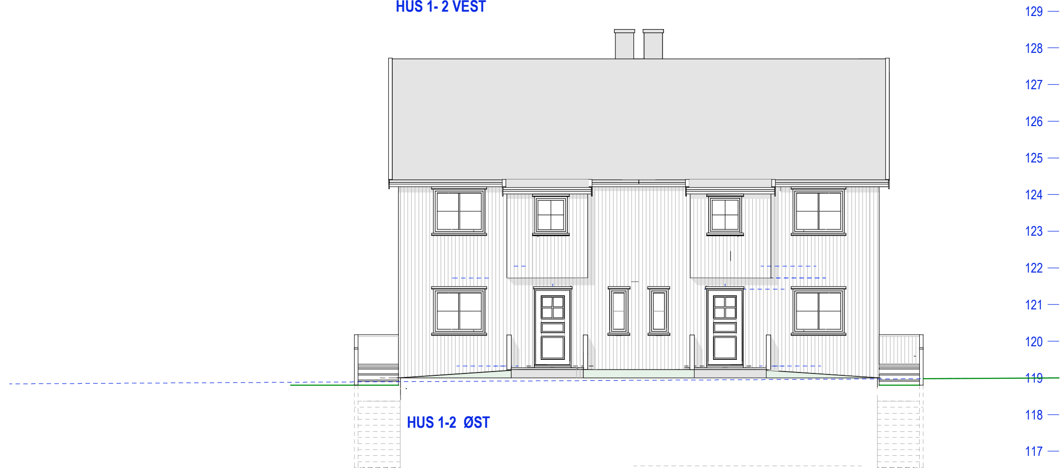
Hus 1-2 E.1-3 Langfasader
