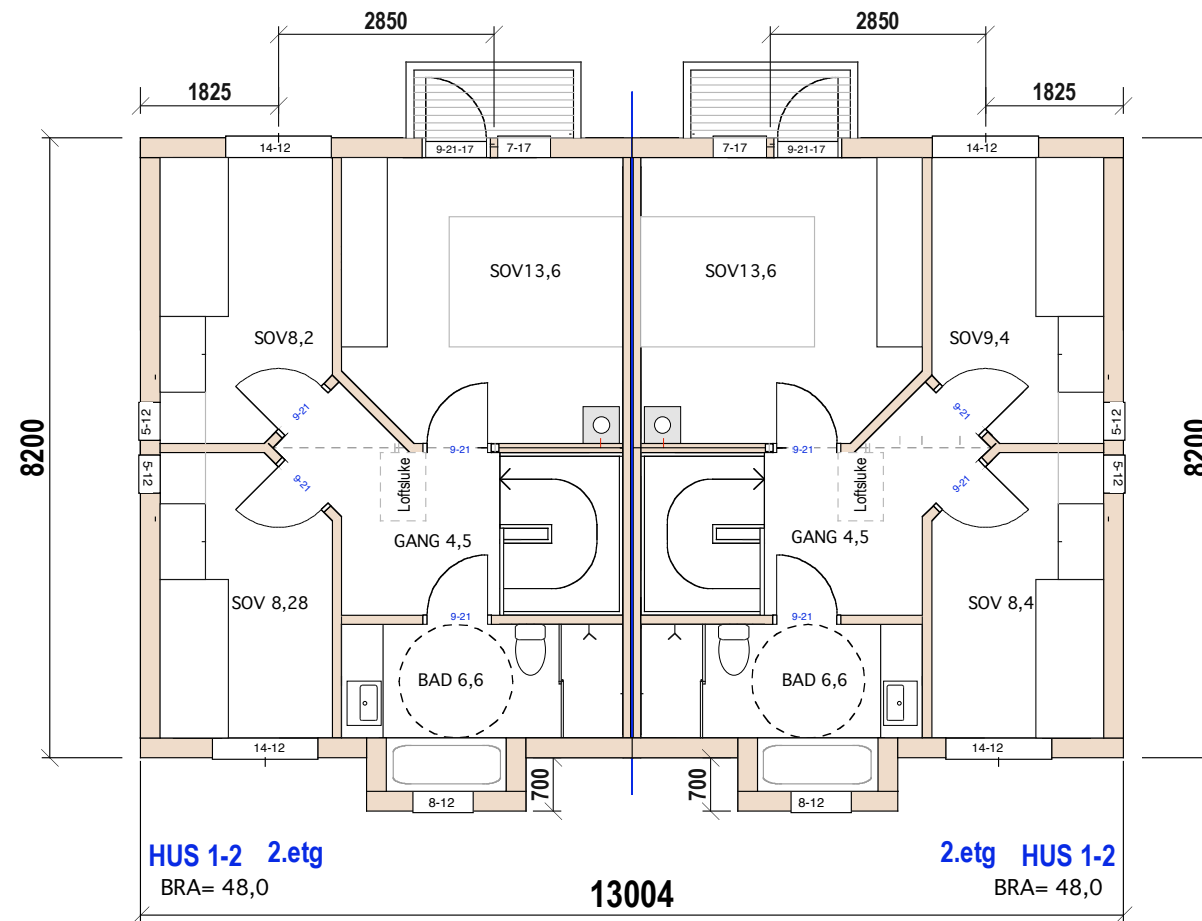
Hus 1-2 E.1-1 Pan 2. etg, loft og snitt
