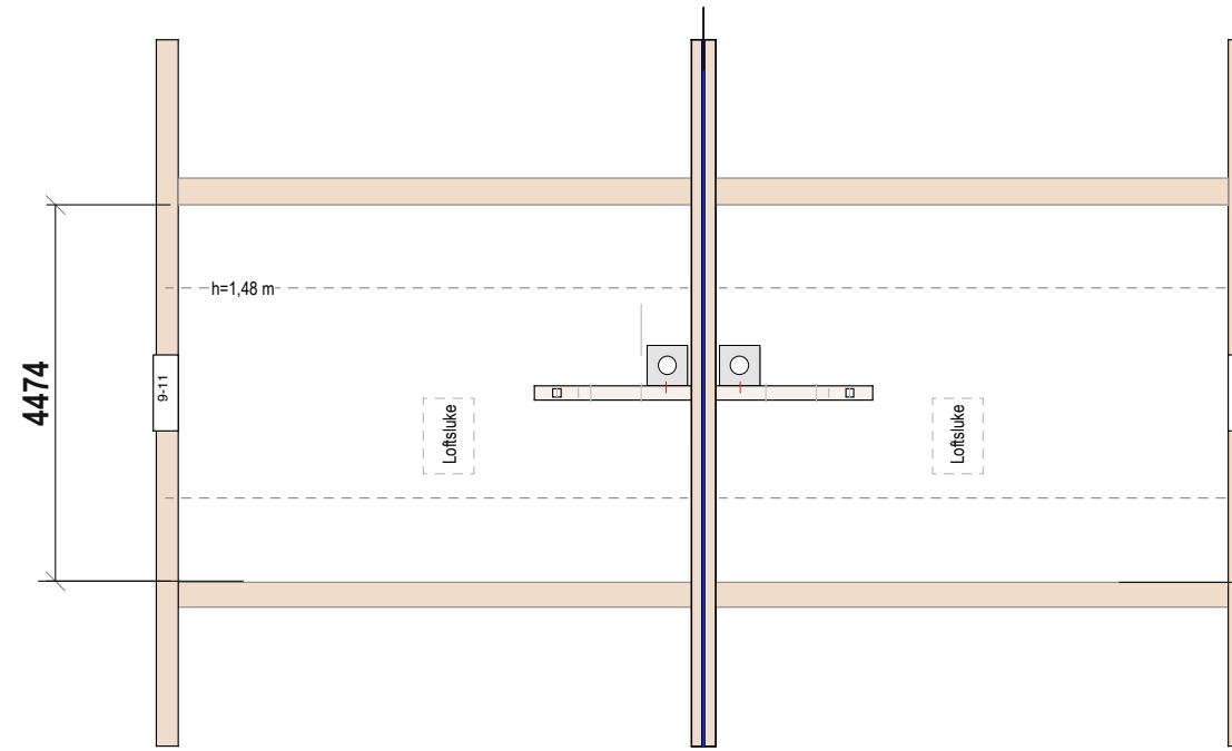
HUS 3-4 Loft
