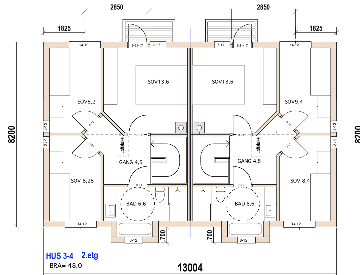
Hus 3-4 E.1-1 Pan 2. etg, loft og snitt
