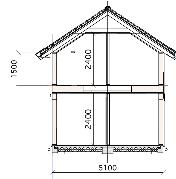
SNITT SIDEBYGG
