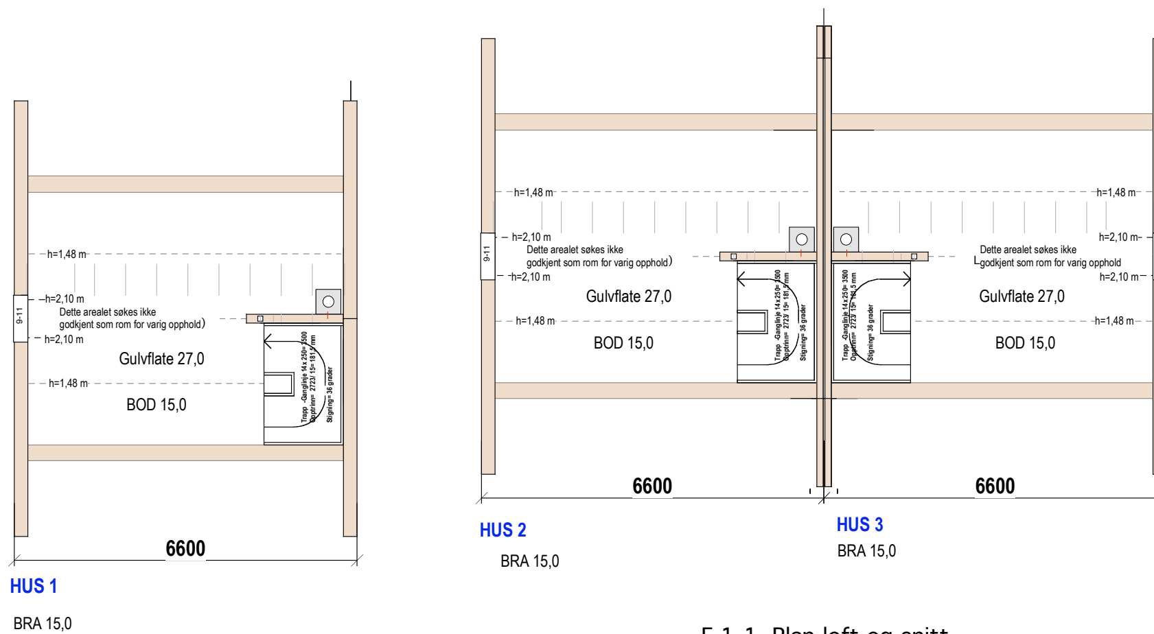
E.1-1 Plan loft og snitt
