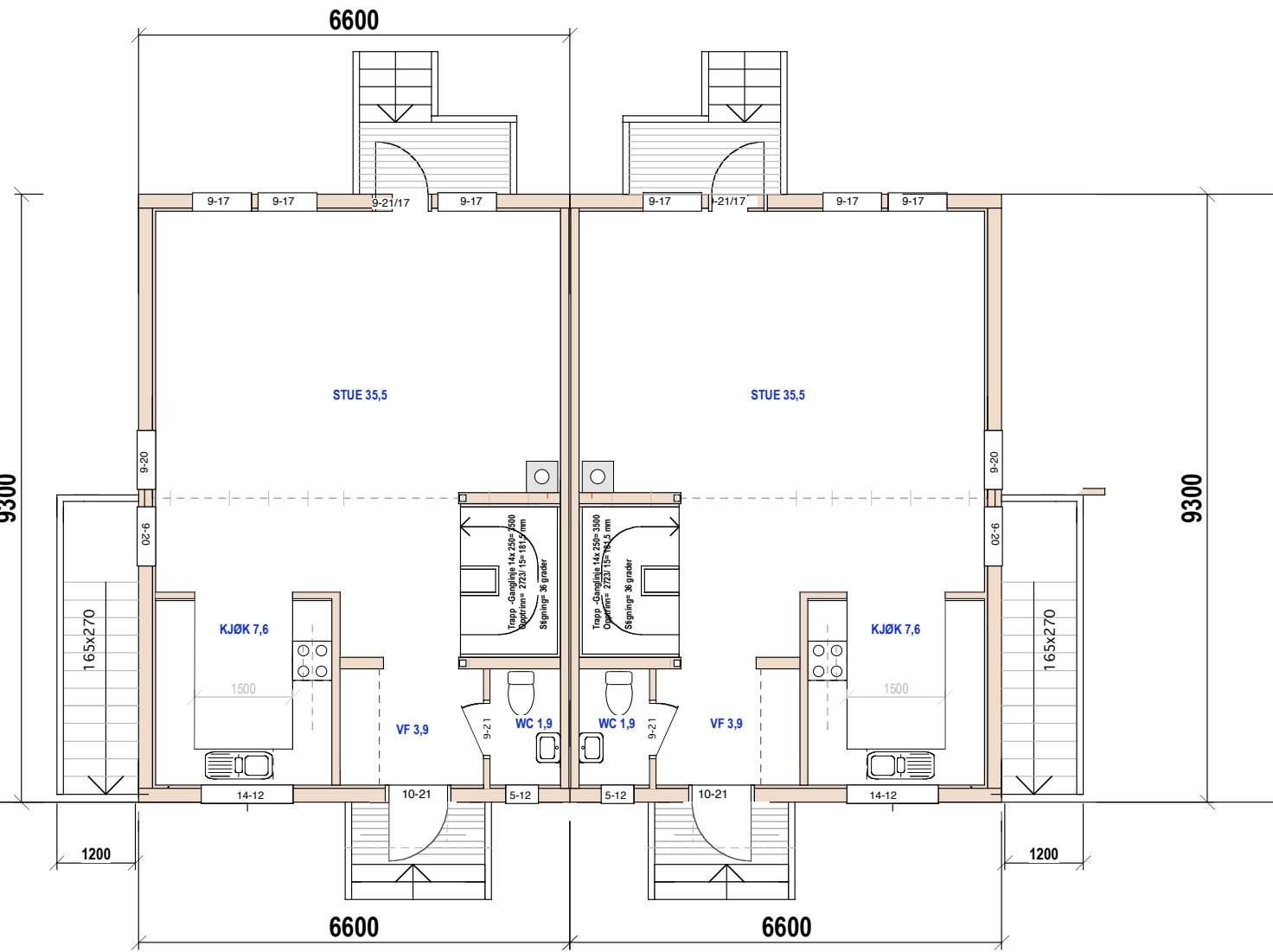
HUS 2 1. etg BRA= 54,5
