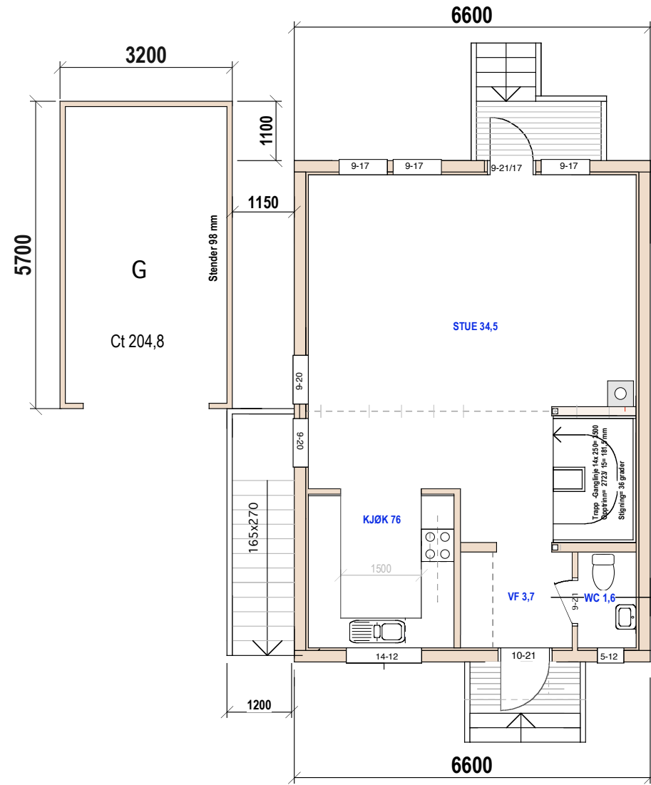
HUS 1 1. etg BRA= 53,5
